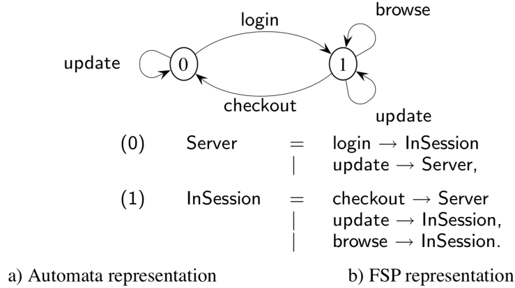
FIGURE 5.1 : Modèle d'une application de base de vente en ligne
