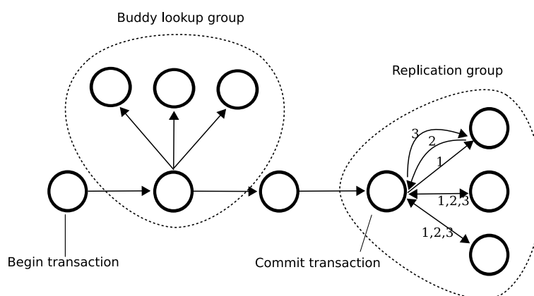
FIGURE 6.4 : Transaction et réplication dans JBoss
