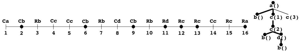
FIGURE 7.2 : Sémantique de path(CallB)
