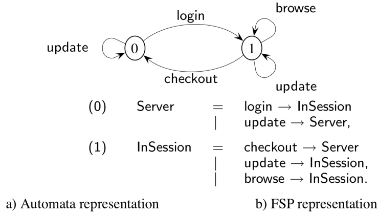
FIGURE 5.1 : Modèle d'une application de base de vente en ligne
