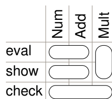
FIGURE 8.15 : Décomposition plus modulaire selon les opérations
