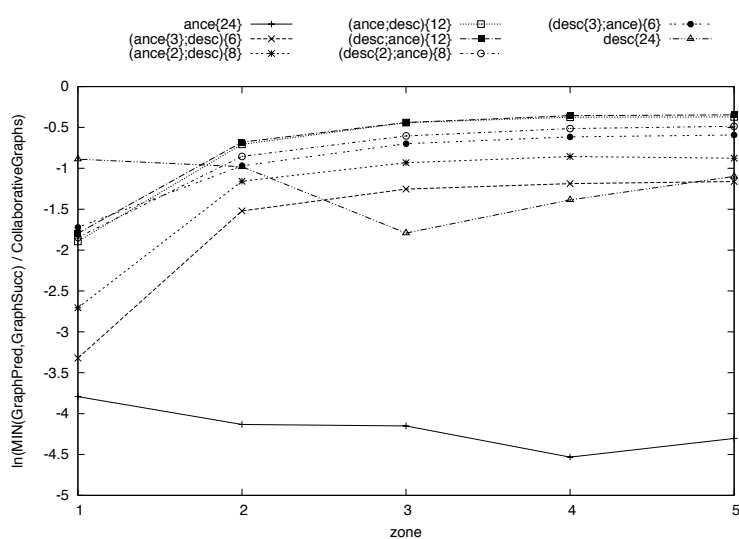
FIGURE 8.9 : Le meilleur de GraphSucc et GraphPred contre notre représentation collaborative
