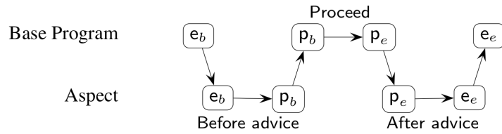
FIGURE 5.4 : Application de vente en ligne tissée par un aspect de cohérence
