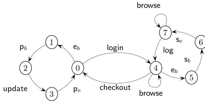
FIGURE 5.5 : Application de vente en ligne tissée par un aspect de cohérence et concurrente
