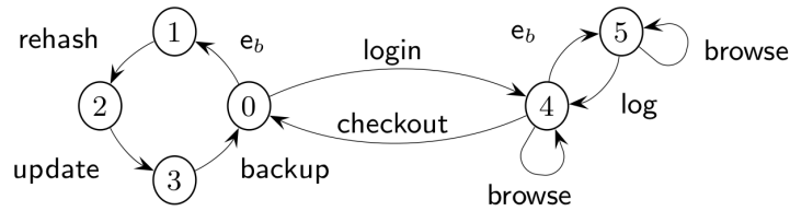
FIGURE 5.6 : L'opérateur de composition Fun pour l'événement e
