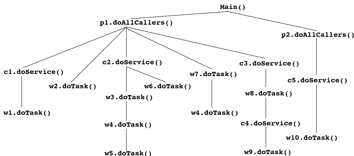
FIGURE 7.3 : Arbre d'appels d'une application à base de clients Caller et services Worker
