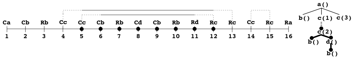
FIGURE 7.1 : Sémantique de cflowBelow(C)
