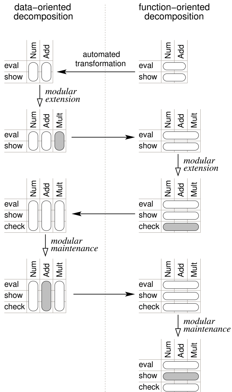
FIGURE 8.16 : Scénario d'évolution
