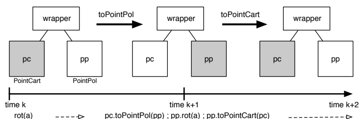
FIGURE 8.1 : Conversion automatique
