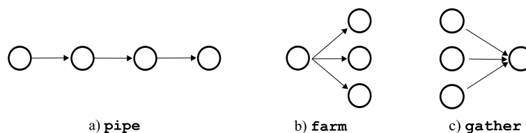
FIGURE 6.5 : Patrons d'interaction
