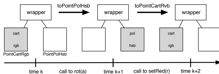
FIGURE 8.3 : Représentations couplées
