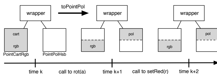
FIGURE 8.4 : Représentations découplées
