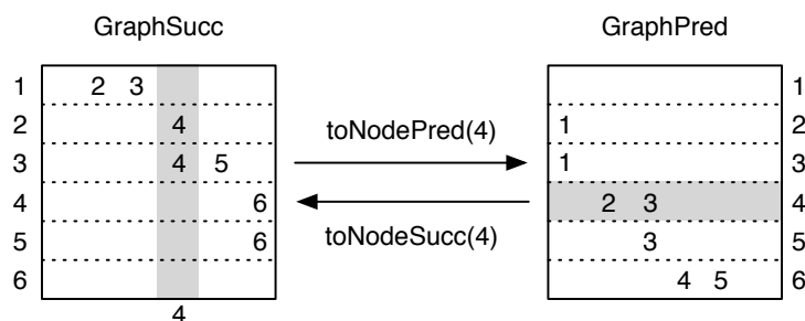
FIGURE 8.8 : Conversion partielle entre lignes et colonnes
