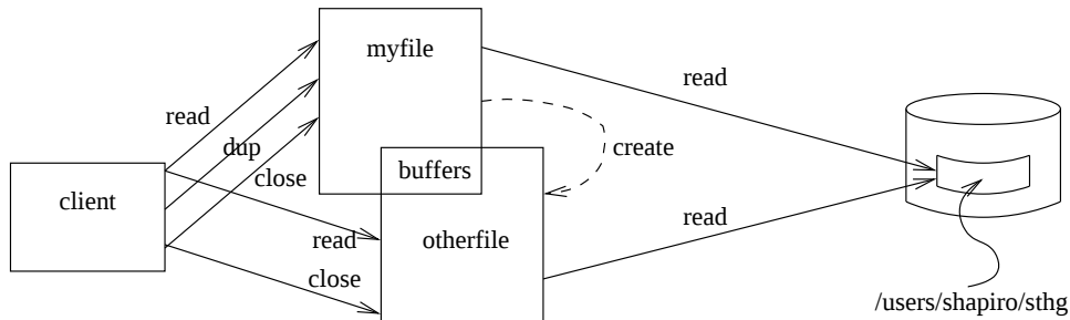
FIG. 2.2 – Fichier accédé comme un objet fragmenté.
