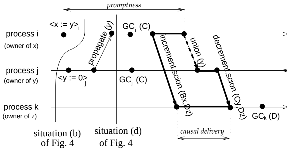
FIG. 4.3 – Effets des règles de sûreté pour l'exemple de la figure 4.2. Sur le site i, l'envoi de increment.scion(B, x, D, z) peut être retardé au plus tard jusqu'à l'envoi de union(y) . Noter la dépendance causale (indiqué par les traits gras) entre les messages increment.scion et decrement.scion , portée par le message union .
