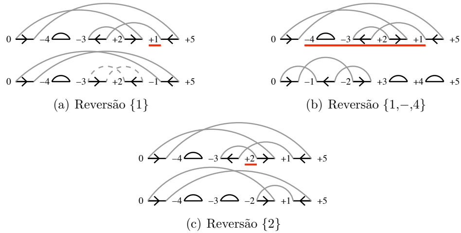
Figura 3.8: A permutação (-4, -3, +2, +1) possui um 4- ciclo orientado com três cruzamentos entre os arcos. O trace \{1\}\{1, -4\}\{2\} agrupa as três reversões que podem ser aplicadas nesta permutação.
