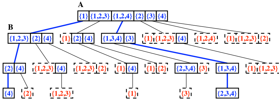
Figura 2.4: Estrutura em forma de árvore que contém os traces que ordenam a permutação \pi = (-3, +2, +1, -4) . Nesta representação, apenas os valores que estão dentro de caixas com bordas sólidas são reversões que efetivamente estão na estrutura. Os valores que estão dentro de caixas com bordas tracejadas são reversões que são optimal 1-sequences mas que, quando adicionadas ao i-trace pai, formam traces que já foram inseridos em outros ramos da árvore. Os dois caminhos com arestas mais largas indicam os traces \{1\}\{1, 2, 3\}\{2\}\{4\} e \{1, 2, 4\}\{3\}\{1, 3, 4\}\{2, 3, 4\} que ordenam a permutação.
