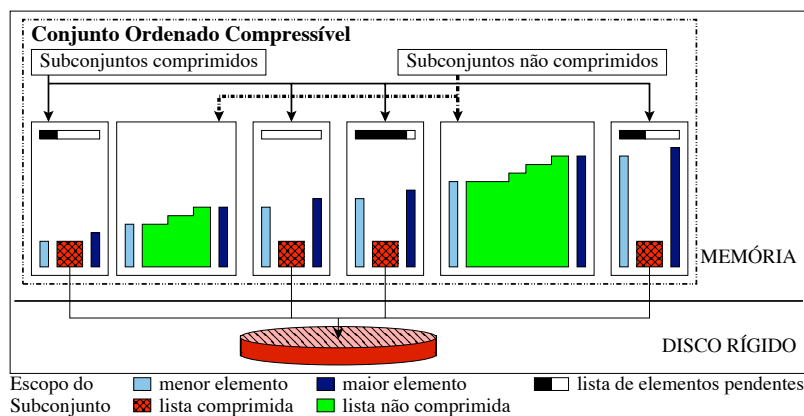
Figura 2.3: Esquema da estrutura “ Compressible sorted set ”. Esta estrutura foi implementada por Braga para gerenciar os dados produzidos durante a execução do algoritmo de enumeração de traces [27,28].
