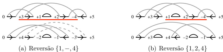
Figura 3.9: A permutação (+3, +1, +2, -4) possui um 4- ciclo orientado com 4 cruzamentos entre os arcos. A primeira sub-palavra do trace \{1, -, 4\} \{1, 2, 4\} \{3, 4\} agrupa as duas reversões que podem ser aplicadas nesta permutação.
