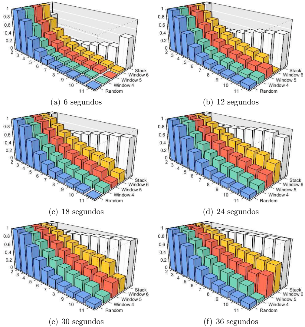
Figura 3.16: Um conjunto de 500 permutações aleatórias com n = 15 e d(\pi) = 12 foram processadas com os algoritmos Random, Window 4, Window 5, Window 6 e Stack utilizando-se diferentes valores de tempo limite (6, 12, 18, 24, 30 e 36 segundos). Para cada trinca (permutação, algoritmo, tamanho médio das reversões contidas no trace ), anotamos a porcentagem de traces que foram encontrados. As barras nos gráficos mostram a média das porcentagens obtidas para cada trinca.
