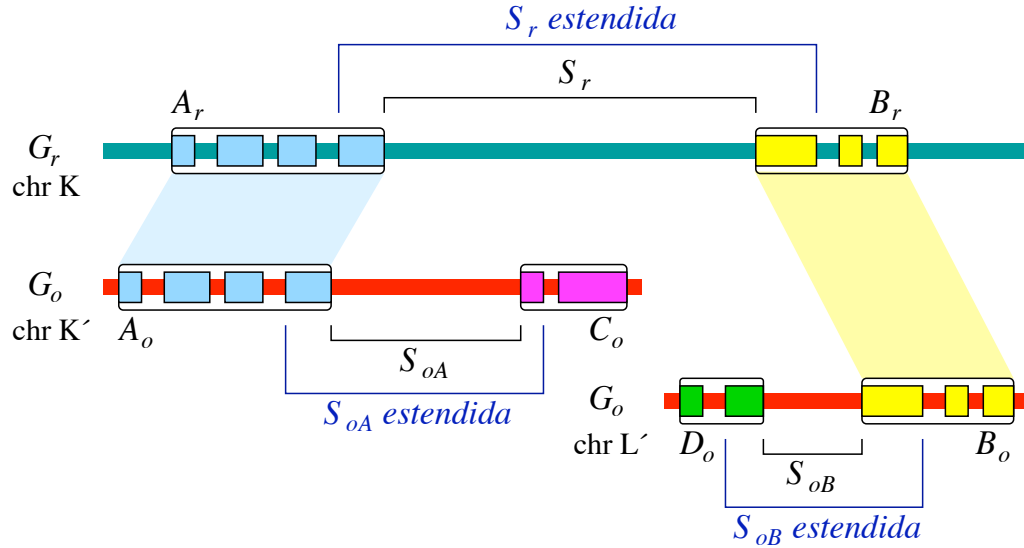
Figura 5.11: Versões estendidas das sequências S_r , S_{oA} e S_{oB} . As versões estendidas destas sequências incluem o primeiro/último gene dos blocos de sintenia que as definem.
