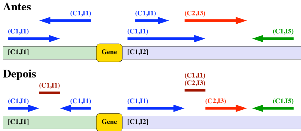
Figura 6.1: Qualquer hit que apresentasse sobreposição com outro foi fragmentado em regiões menores para distinção de locais que são cobertos por um único hit e locais que são cobertos por múltiplos hits (que diferem ou em relação ao par (C_o, I_o) ou em relação à orientação \sigma_o ).
