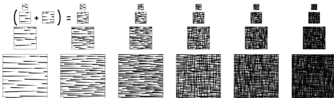
FIG. 2.5: Tonal Art Map de Praun et al. (74). Les hachures d'une image apparaissent dans toutes celles qui la suivent en dessous ou à sa droite.
