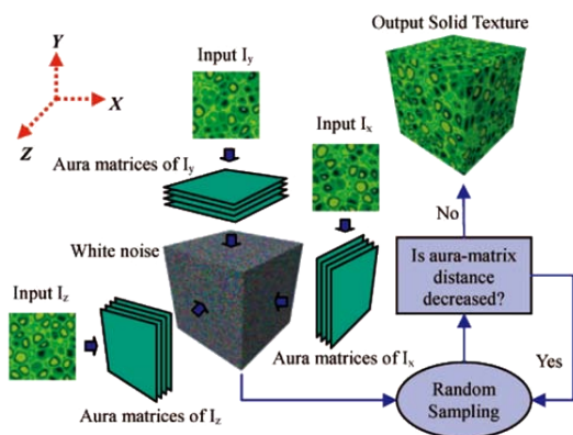
FIG. A.4: Principe schématisé de l’algorithme de synthèse de Qin et Yang (77).
