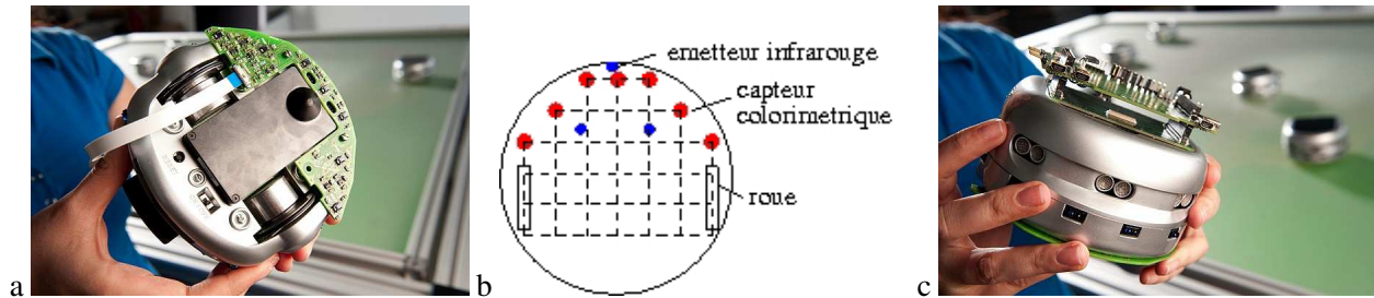
FIGURE 3 – Photos d'un robot Khepera III et de ses cartes d'extension pour interagir avec la Table. a) capteurs colorimétriques et émetteurs infrarouges. b) schema de la position des capteurs et emetteurs. c) carte arduino et d'acquisition.
