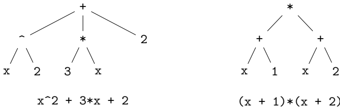
FIGURE 2.1 – Deux expressions symboliques qui représentent le même objet mathématique.
