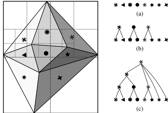
Figure 4: Construction de la hiérarchie : à gauche, l'objet plongé dans un octree avec une face (son centre) par cellule ; à droite, (a) les centres correspondant aux feuilles de l'octree ; (b) après une itération de la reconstruction ; (c) la hiérarchie correspondant à l'objet.
