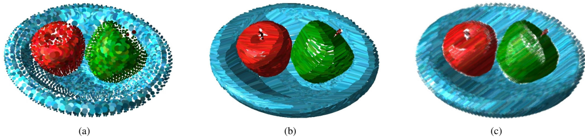
Figure 6: Différents exemples de styles d'une même scène : (a) Pointilliste en variant la taille en fonction de l'angle entre la normale et le point de vue ; (b) l'orientation des coups de pinceau est modifiée par la normale des objets pour mieux faire ressortir la forme, la couleur provient d'un toon shading ; (c) ici l'orientation des coups de pinceau est constante, on notera ici la bonne représentation des dégradés.
