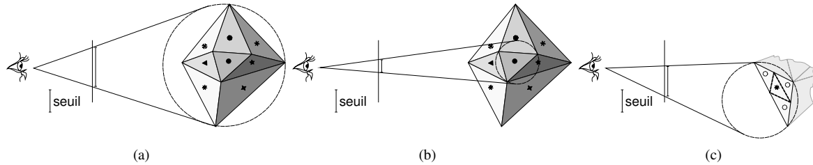
Figure 5: Sélection des points d'attache : (a) la projection de l'objet est trop grande pour être représentée par un seul coup de pinceau ; (b) on descend donc dans la hiérarchie jusqu'à atteindre un noeud de taille convenante ; (c) si on atteint une feuille de la hiérarchie trop grande, on la subdivise dynamiquement.
