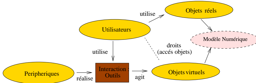
FIG. 3 – Modèle de gestion de l'interaction entre l'utilisateur et les objets réels et virtuels.
