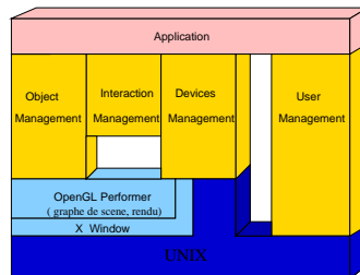
FIG. 4 – Architecture logicielle de notre système découpé en modules. La mise en oeuvre repose sur le langage C++, qui nous permet d'utiliser les avantages des langages objet.
