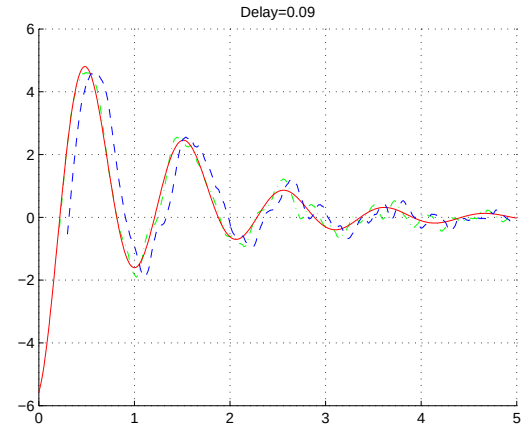
(d) Affine causal estimator \hat{x}_{t_0-}(k, \mu, -T, 2, \xi)
