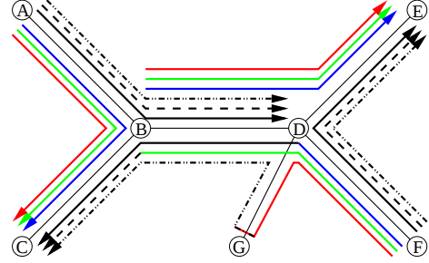
FIG. 1: Chemin non-simple de F à C dans un réseau à 1 fibre, 6 couleurs et au plus 1 conversion par sommet.
