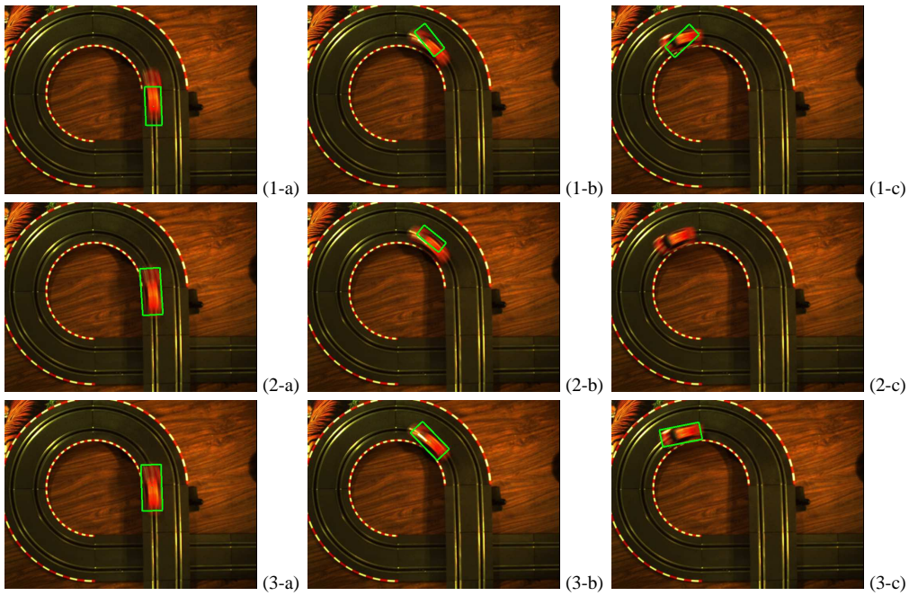
FIG. 5 – Résultats comparatifs des différentes approches avec des translations, rotations et changement d'échelle. 1e ligne : filtre particulaire avec 1 noyau, et 500 particules. 2e ligne : approche déterministe multi-noyaux [8]. 3e ligne : filtre particulaire avec 9 noyaux constants, et 500 particules.
