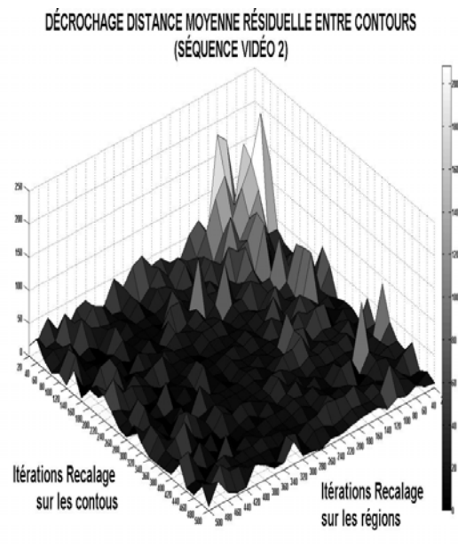
Figure 13: Nombre de décrochages de la distance moyenne résiduelle entre contours (l'axe vertical) par rapport au nombre d'itérations de recalage sur les régions et de recalage sur les contours (axes horizontaux) obtenue sur la séquence vidéo 2. Les expérimentations sur les séquences vidéo 1, 3, 4, 5 et 6 donnent des résultats similaires.
