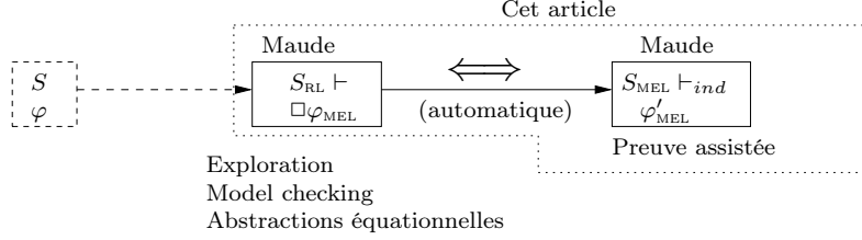
FIGURE 1 – Notre approche dans le contexte des outils de vérification du système Maude.
