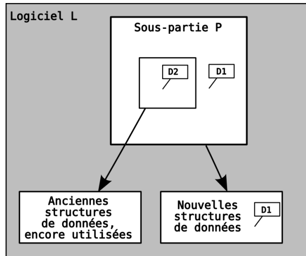
FIGURE 1 – Situation du code juste après la fusion des deux développements réalisés en parallèle. On souhaite que le code du développement D_2 utilise maintenant les nouvelles structures de données comme le reste de la partie P du logiciel.
