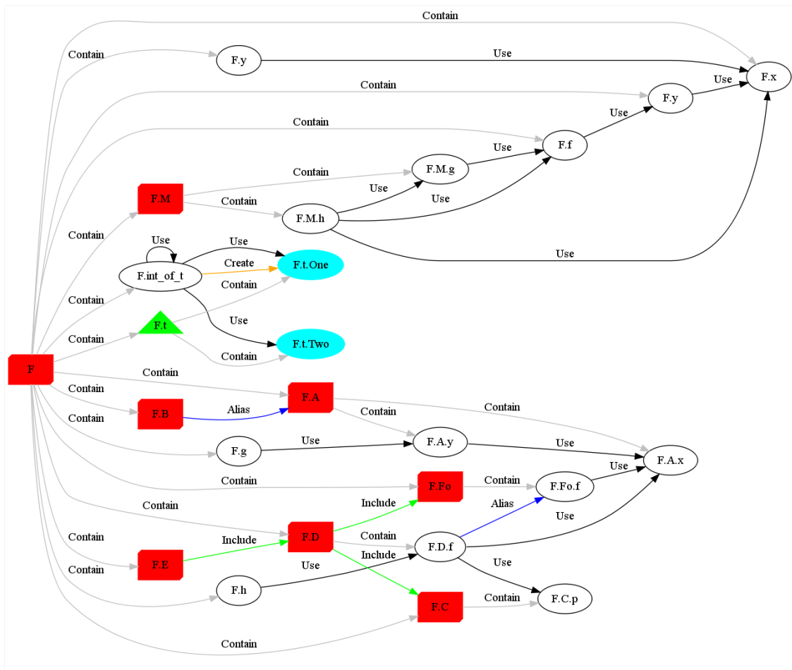
FIGURE 5 – Graphe annoté des éléments exportables de l'exemple.
