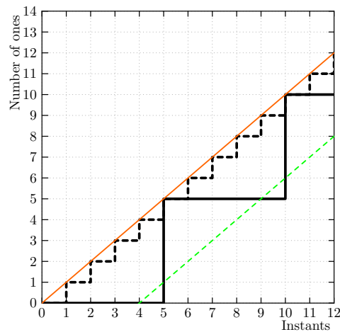
FIGURE 7 – Modélisation de la lecture/écriture de plusieurs valeurs au sein du même instant
