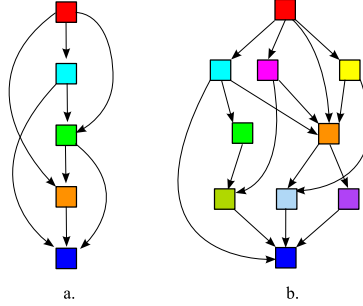
Figure 3: a. a linear DAG. b. a non-linear DAG
