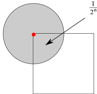
FIG. 2.10 – Cas le plus défavorable : notre requête est proche d'un coin de la cellule, en dimension n . Seul 1/2^n -ième de la boule de plus proche voisins est récupéré : la dimension dégrade le rappel de façon exponentielle.
