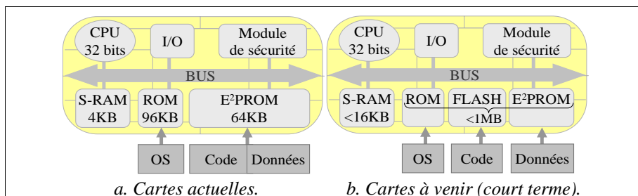
Figure 1. Architectures des cartes à puces.
