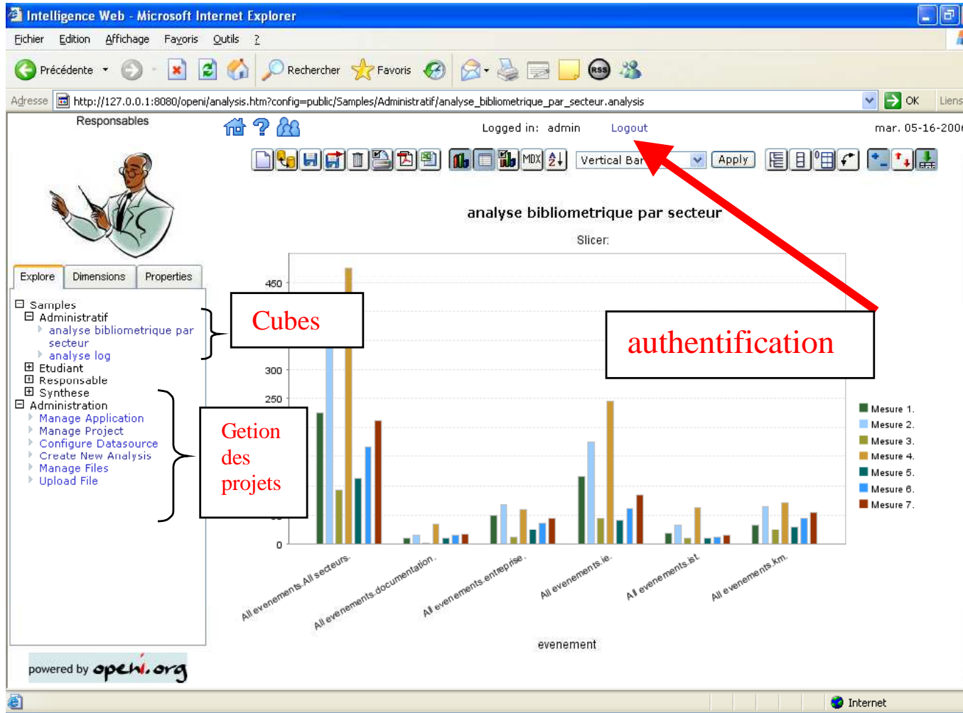
Figure 2 : Environnement graphique d'analyse et de gestion d'Openi
