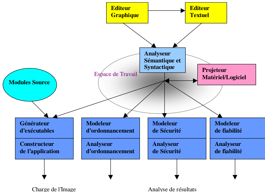
Figure 6.1 : Environnement MetaH
