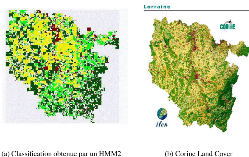
Figure 10. Classification obtenue par un HMM2 à 10 états après 10 itérations et comparaison avec la carte de la Lorraine établie dans le cadre du programme Corine Land Cover à partir de données satellitaires (IFEN, 1993)
