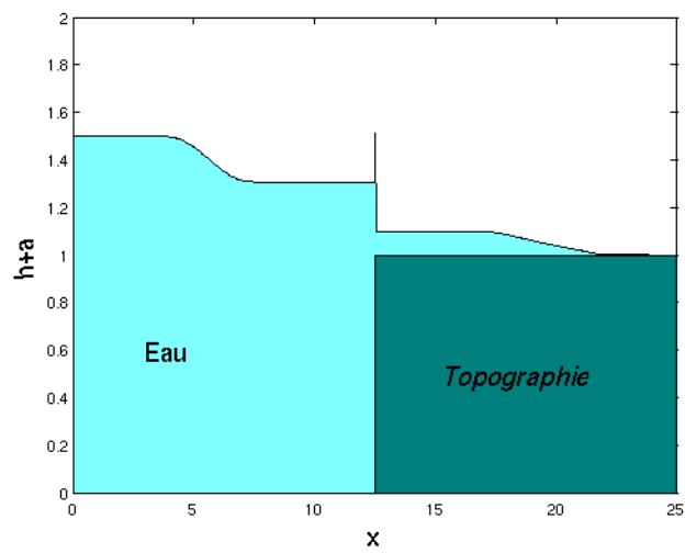
FIG. 13 – Test4 ( t=2s )
