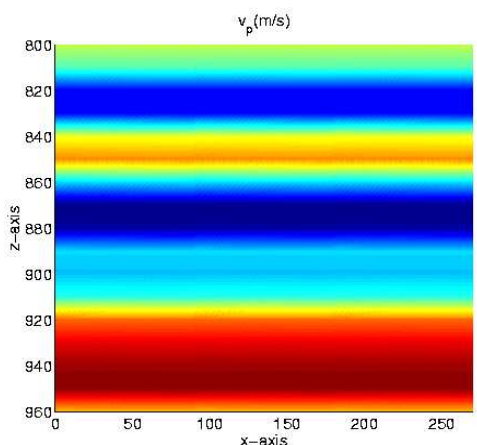
FIG. 27: Vitesse des ondes P
