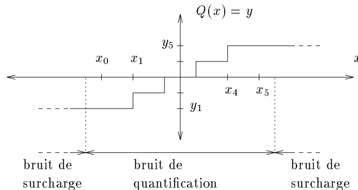
FIG. 3 - Exemple d'un QS uniforme pour L = 5
