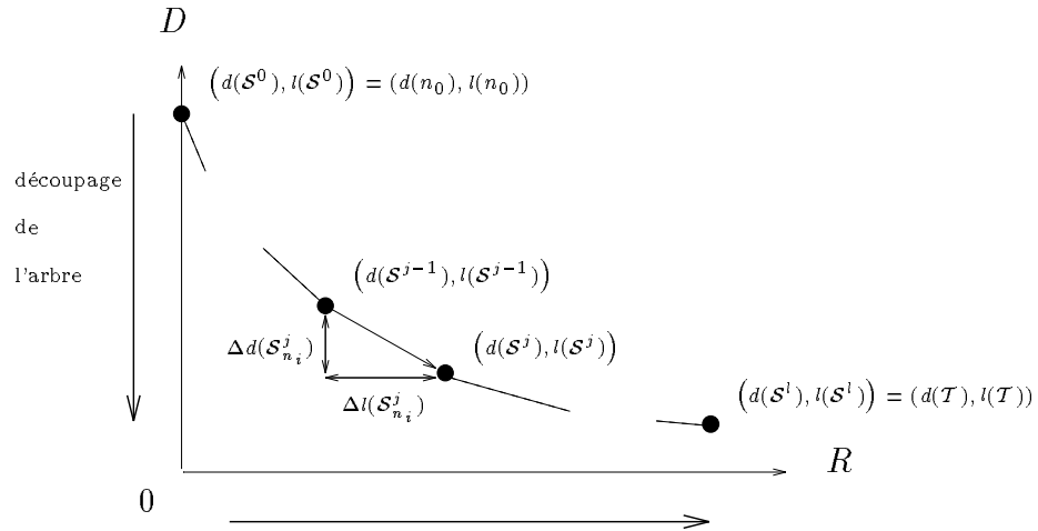
FIG. 38 - Découpage de l'arbre : cas où, à l'itération j de l'algorithme, la branche \mathcal{S}_{n_i}^j est ajoutée.
