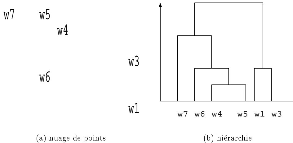
FIG. 1.2 – Classification hiérarchique
