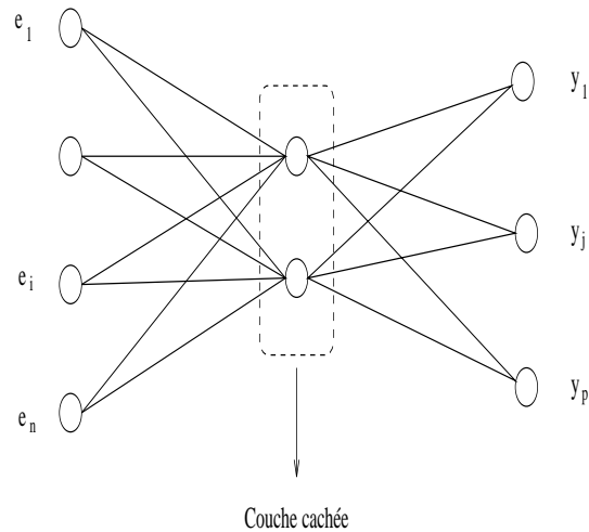
FIG. 3.5 – Perceptron multicouche
