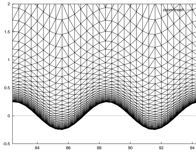
FIG. 23 - Cas 2 : zoom du domaine : 14 eme et 15 eme rugosités
