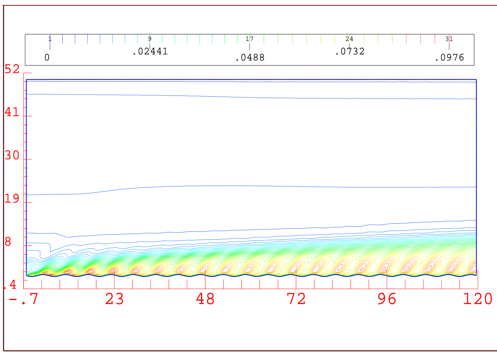
FIG. 22 - Cas 2 : isovaleurs de \sqrt{\frac{2k}{3}}
