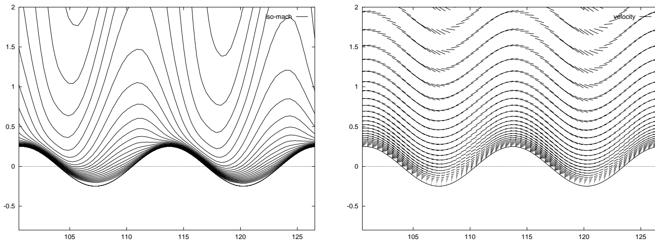
FIG. 12 - Cas 1 : Zoom : iso-mach (gauche) et champ de vitesse (droite).
