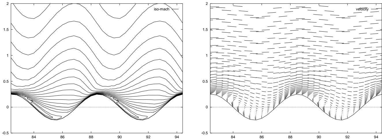
FIG. 24 - Cas 2 : Zoom : iso-mach (gauche) et champ de vitesse (droite)
