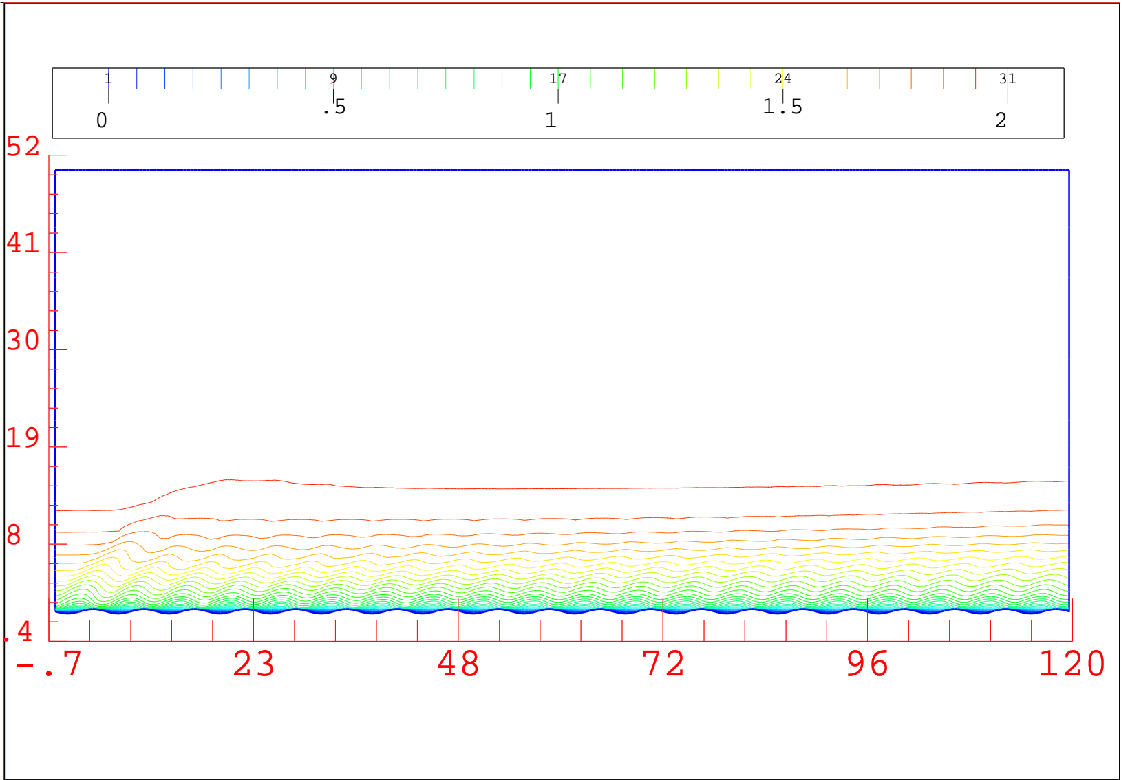
FIG. 19 - Cas 2 : iso-mach
