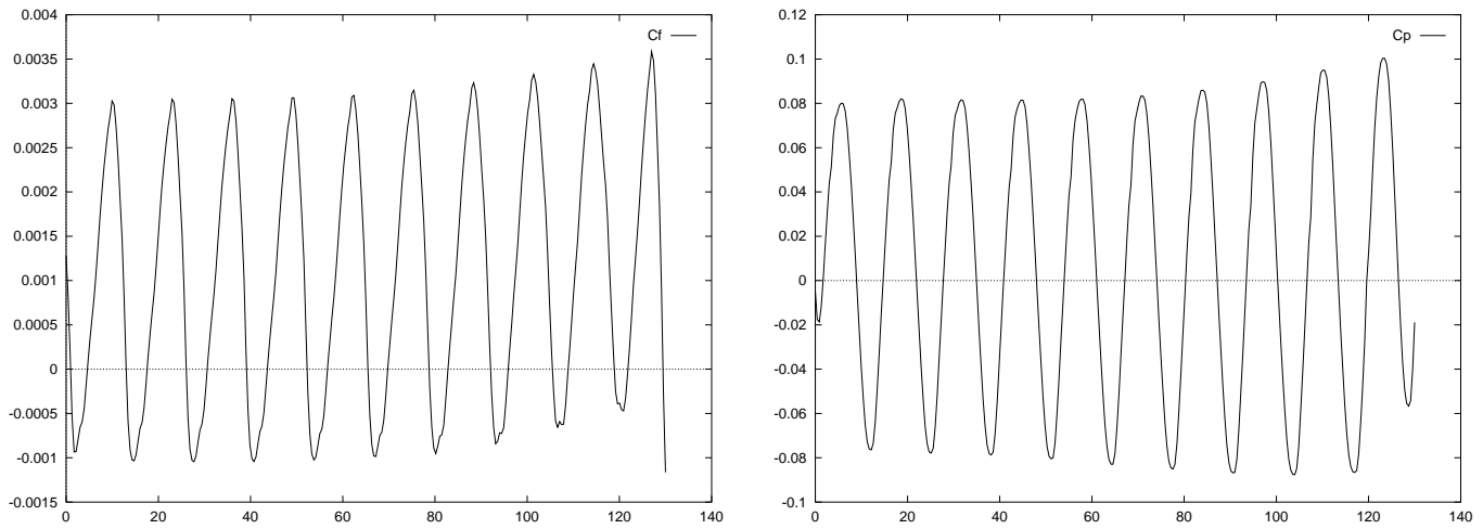
FIG. 7 - Cas 1: C_f (gauche) et C_p (droite).
