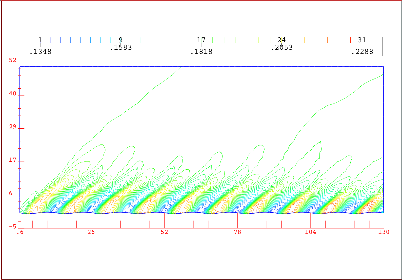
FIG. 8 - Case 1 : iso-pressure.
