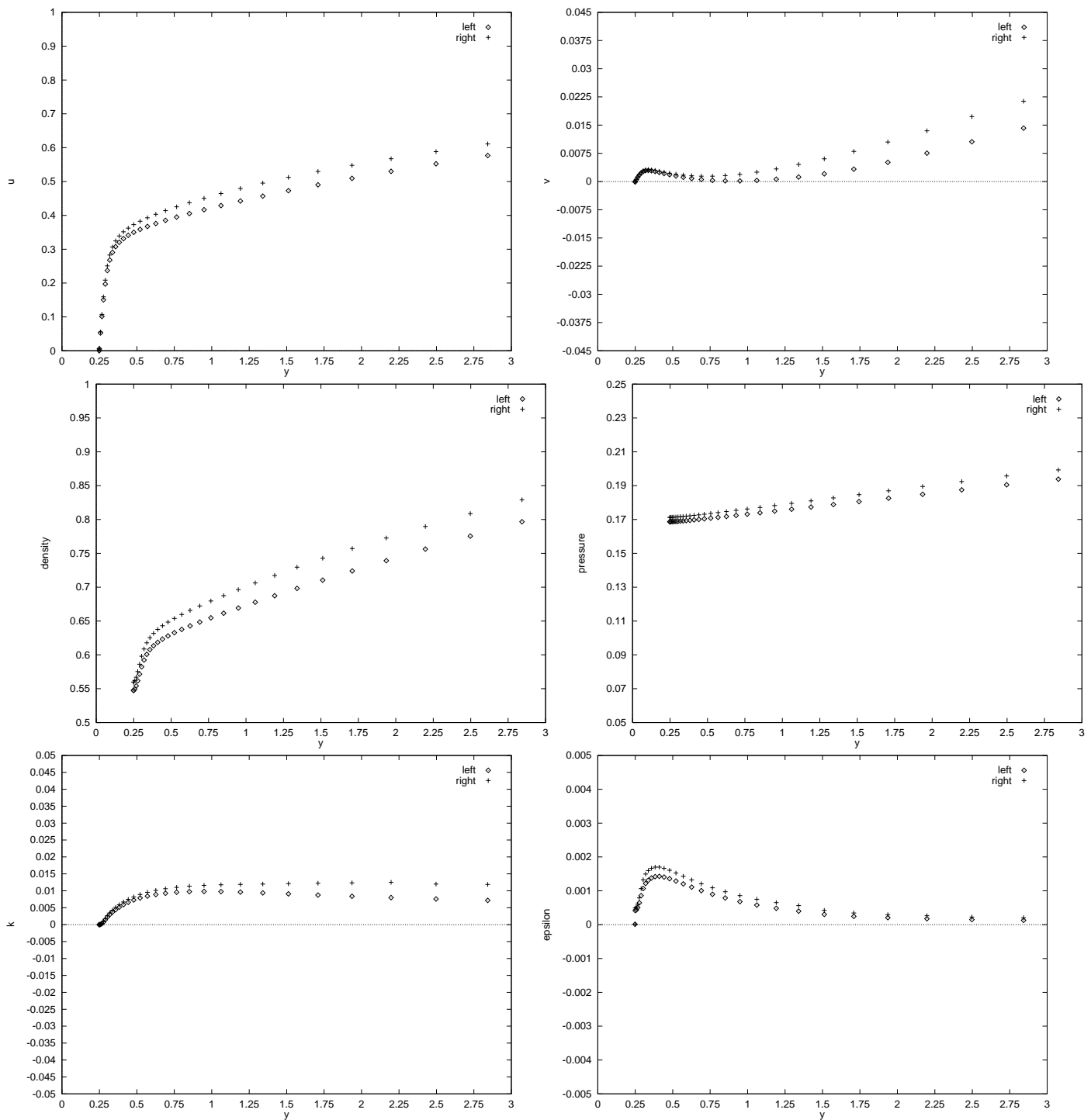
FIG. 13 - Cas 1 : Comparaison du profil entre deux rugosités : vitesse tangentielle, vitesse normale, densité, pression, énergie turbulente et dissipation de l'énergie turbulente. Ici, y correspond à y = y + \frac{h}{2} .
