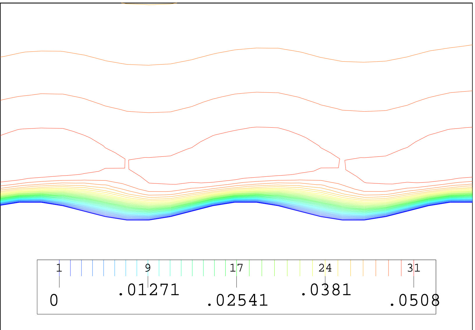
FIG. 39 - Cas 3 : zoom des isovaleurs de \sqrt{\frac{2k}{3}} avec bicouche, 14 eme et 15 eme rugosités
