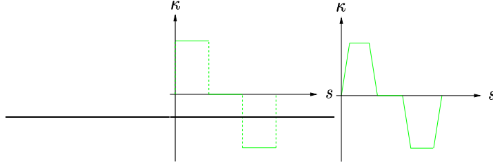
FIG. 3 – profils de courbure (Dubins / CSCC).
