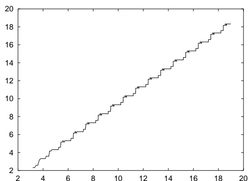
n_0 = 8
