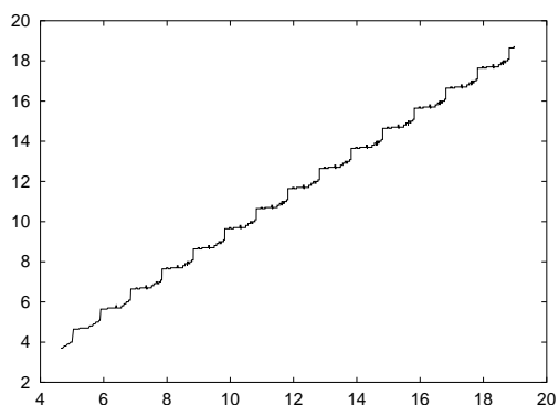
n_0 = 24
