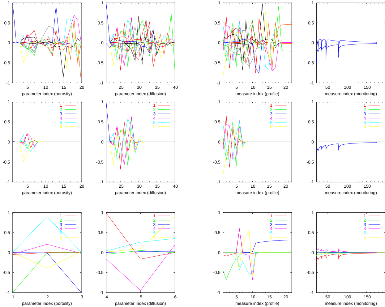
FIG. 6.16 – Vecteurs singuliers en un point correspondant à une modification de la porosité et du coefficient de diffusion du milieu de référence. En haut, au milieu : dans le cas de la paramétrisation fine à 20 zones (vecteurs singuliers associés aux 21 valeurs singulières au-dessus du niveau de bruit, puis associés aux 6 premières valeurs singulières), en bas : dans le cas de la paramétrisation grossière à 3 zones. À gauche : dans l'espace des paramètres, à droite : dans l'espace des mesures.
