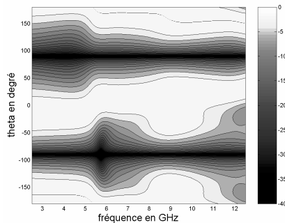
Figure 4 : Diagrammes de rayonnement (niveau en dB), plan E, en fonction de la fréquence, triplaquée.
