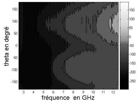
Figure 6 : Diagrammes de phase, plan E, en fonction de la fréquence, triplaquée.
