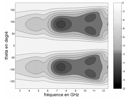
Figure 5 : Diagrammes de rayonnement (niveau en dB), plan H, en fonction de la fréquence, triplaquée.
