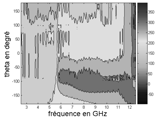
Figure 7 : Diagrammes de phase, plan H, en fonction de la fréquence, triplaquée.
