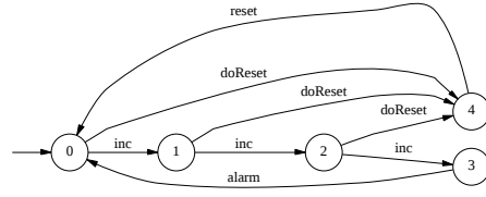
Fig.3. Modèle du compteur du TC
