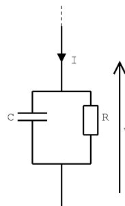
Fig. 3 : Circuit électrique équivalent au neurone I&F
