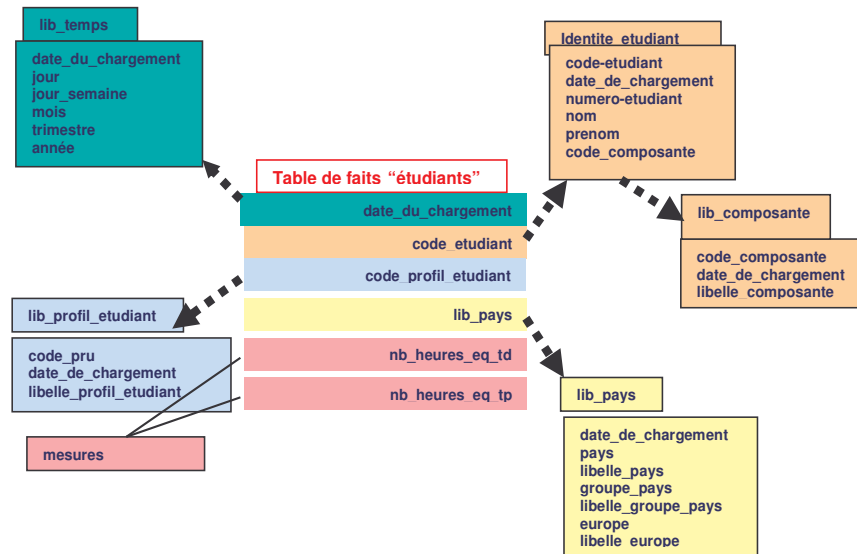
Figure 5 - Schéma en flocon de neige
