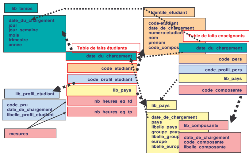
Figure 6 - Constellation de faits
