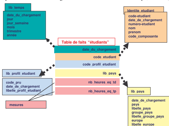
Figure 4 - Schéma en étoile
