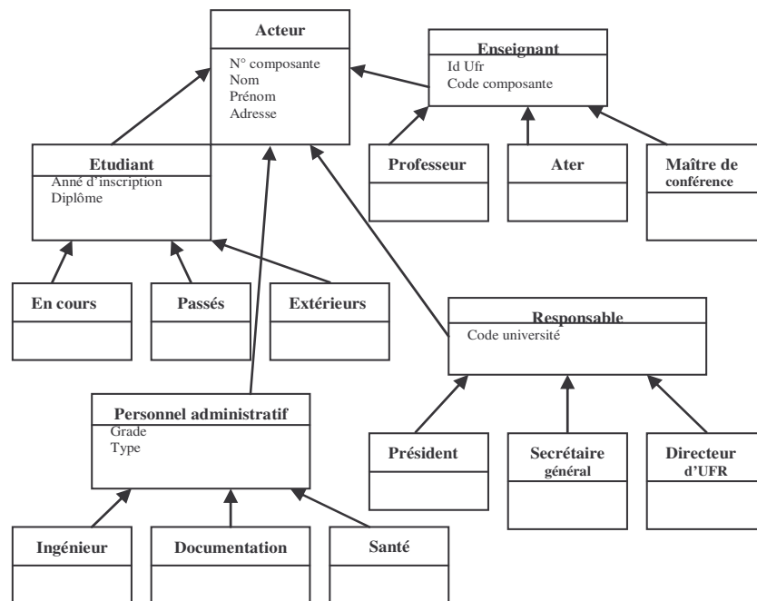
Figure 9 - Modélisation des types d'acteurs
