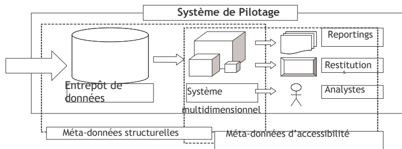
Figure 18 – Méta-données structurelles et d'accessibilité
