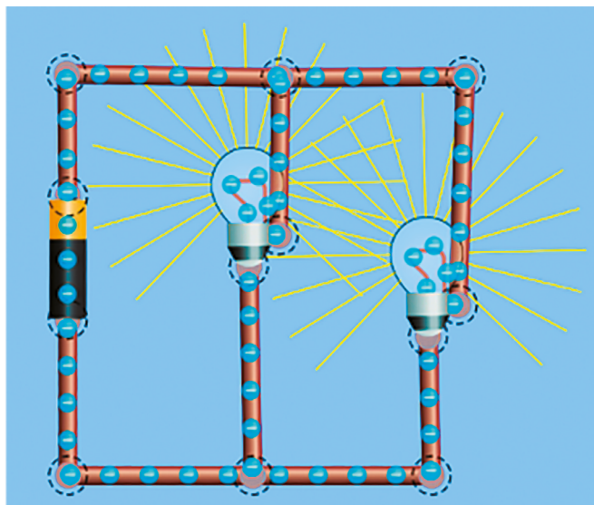
→ Montage en dérivation
