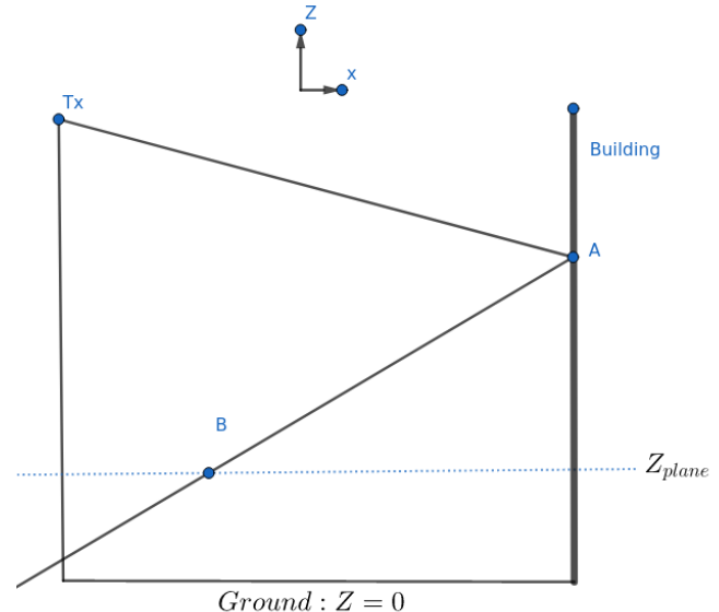
Fig. 2. Ray-plane intersection
