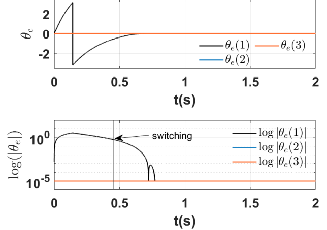
Fig. 1. Rotation error \theta_e
