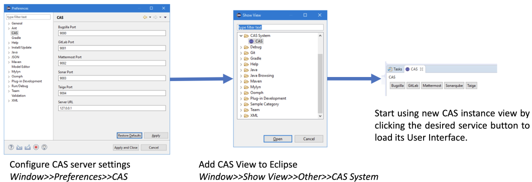
Fig. 2. Configuring CAS
