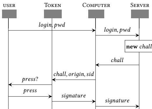
Fig. 4. U2F protocol
