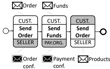
Fig. 2. BPMN Choreographie [28]
