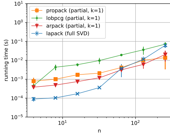
(d) SVD for matrices of size n \times n
