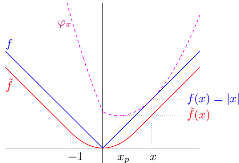
Fig. 3.10. Régularisée de Moreau-Yosida \tilde{f} de f : x \mapsto |x|
