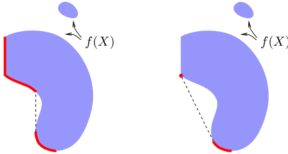
Fig. D.1. Image par f des points Pareto optimaux (g) et moyennement optimaux (d)
