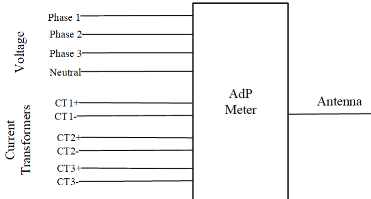
Fig. 6. AdP meter interfaces
