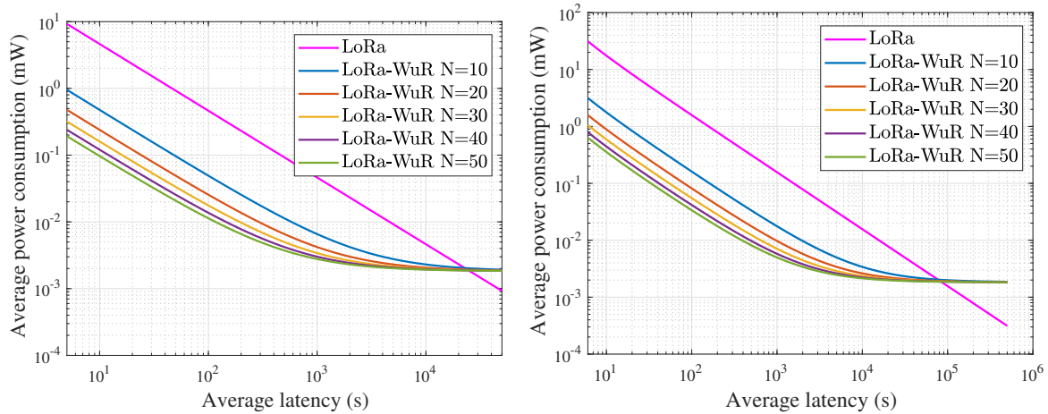
(a) Config. 1: SF=6 , BW=500KHz , CR=\frac{4}{5}
