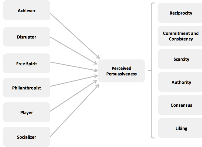
Fig. 2. PLS-SEM Model
