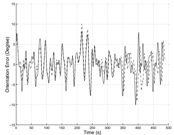
Fig. 4. Orientation error
