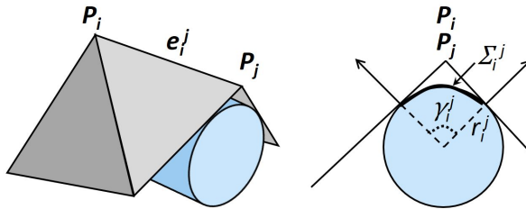
FIGURE 1.4 – L'arête e_i^j entre le sommet P_i et un sommet voisin P_j est approximée par la portion cylindrique tangente \Sigma_i^j de rayon r_i^j .
