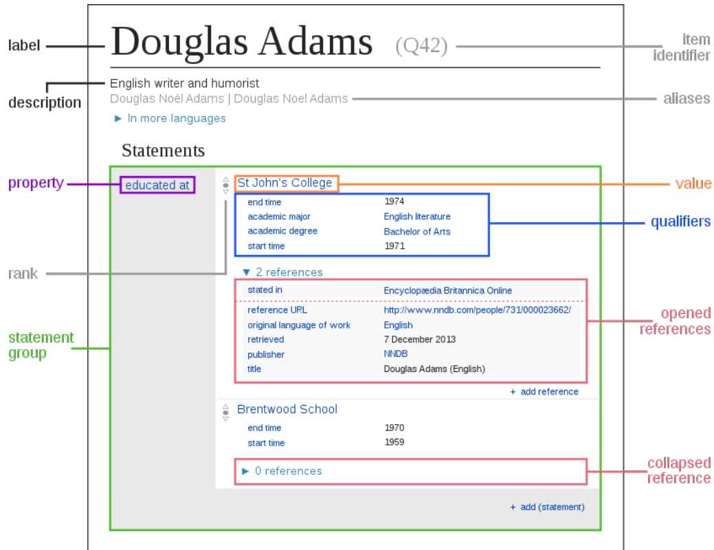
Figure 4. Data model in Wikidata
