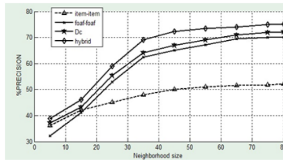
Fig. 3. Precision rate
