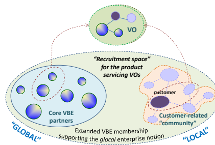
Fig. 3 – Extended VBE
