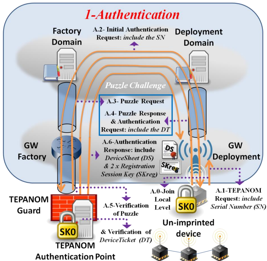
Fig. 3. TEPANOM Authentication Phase.
