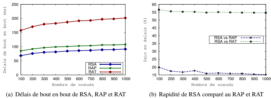
Figure 8 – Délai de bout en bout
