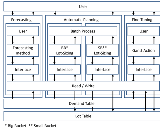
Fig. 1. OOPUS WEB Task Model
